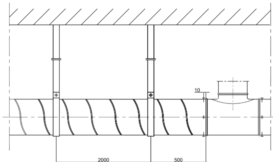
Joonis 1 Paigaldusjoonis
