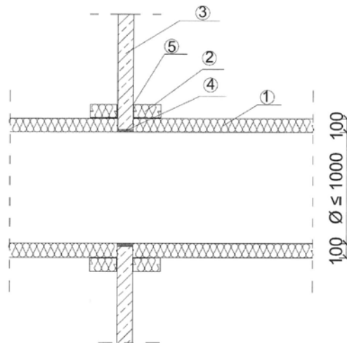
Joonis 3b. CONLIT MAT võrkmatiga isoleeritud ventilatsioonikanali läbiviik betoon- või tellisseinast:
