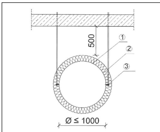
Joonis 2. Ventilatsiooni õhukanalite paigaldamine, läbilõige riputuselemendi kohal: 1 – õhukanal; 2 –CONLIT MAT võrkmat; 3 – õhukanali riputuselement, mis koosneb standardsest hoidikust ja mutritega tikkpoldist.
